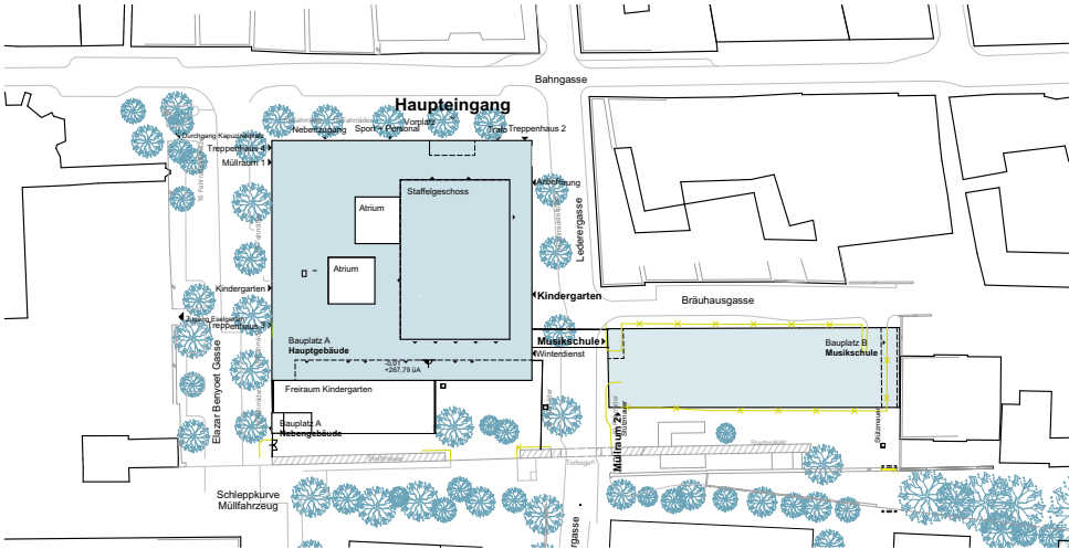
Lageplan site plan
