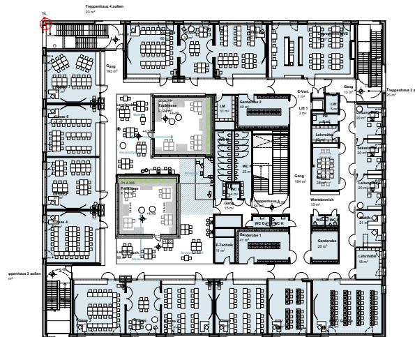
1. Obergeschoss first floor
